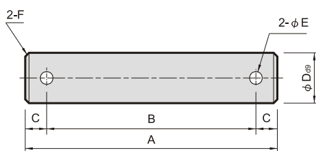
CA & CB 型兩種裝配型式插銷尺寸表：
